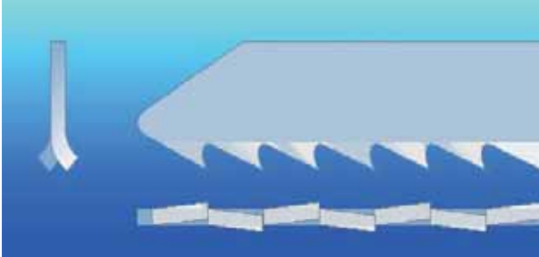
Geschränkte Zahnung
